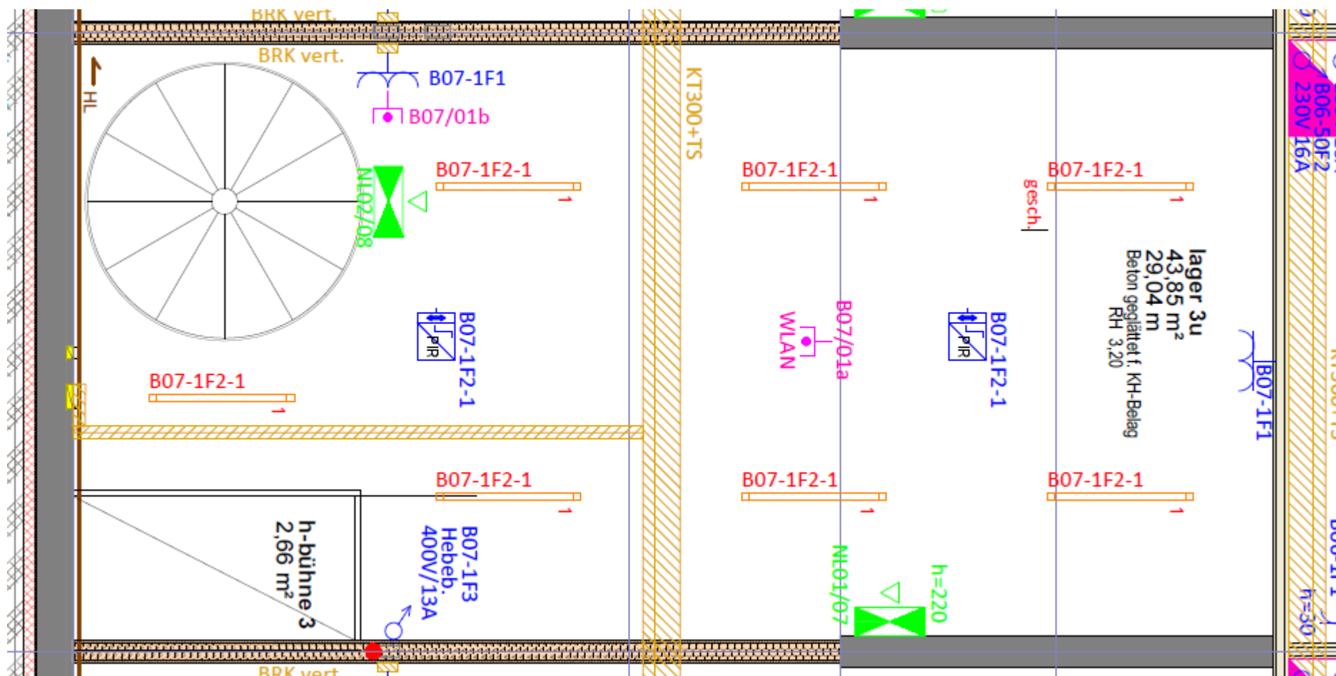
Abbildung 3: Grundriss Untergeschoss
