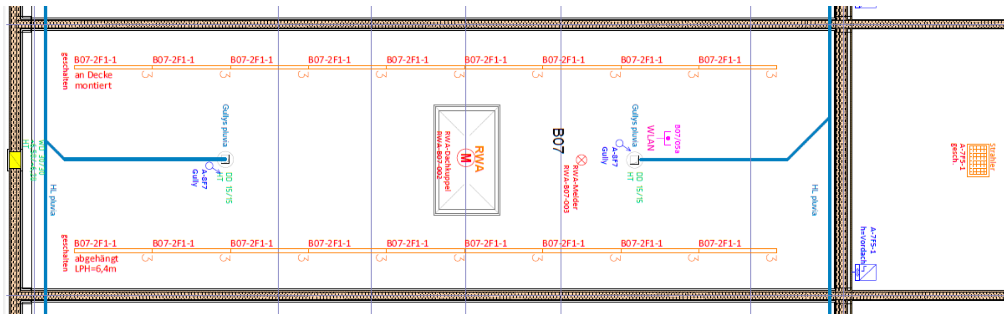
Abbildung 1: Grundriss Erdgeschoss (Decke)
