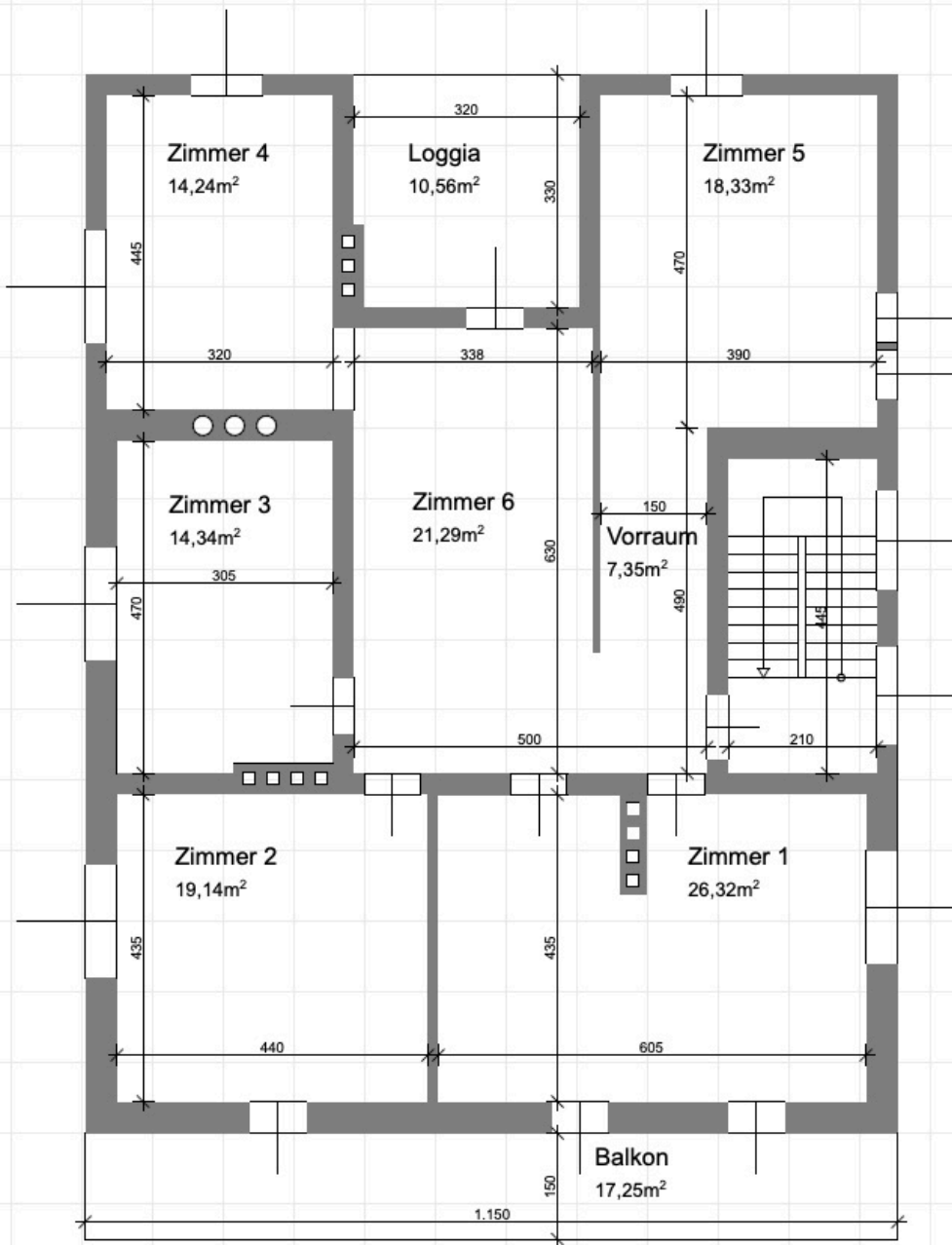
1.Obergeschoss
