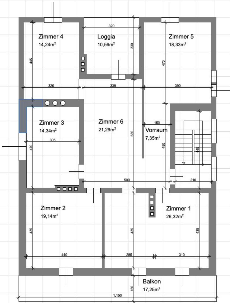
2.Obergeschoss
