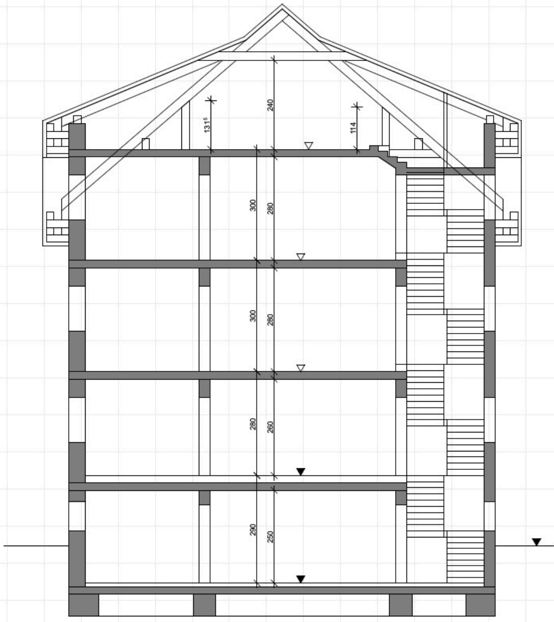
Querschnitt
